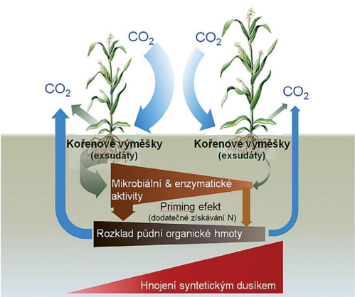
Obr. 2 Změny interakcí mezi rostlinami, mikroorganismy a půdou při zvyšujícím se přísunu dusíku ve formě syntetického dusíkatého hnojení (vysvětlení v textu). Šířka šipek odpovídá intenzitě procesů. Upraveno podle Kumar et al., (2016).
